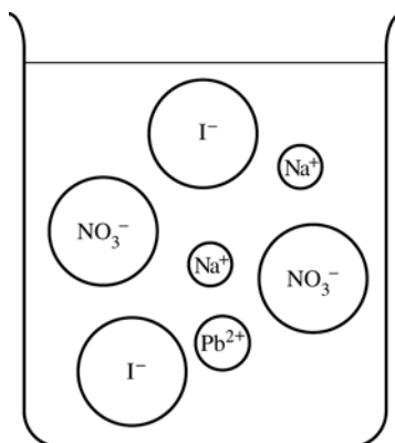
No Precipitate
